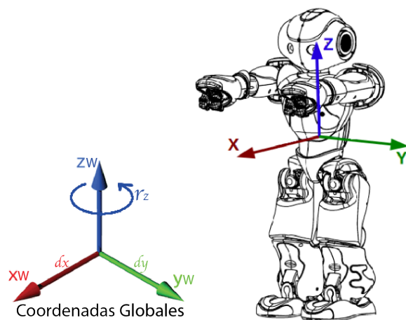
Figura 4.2: Sistema de Coordenadas del Robot NAO
